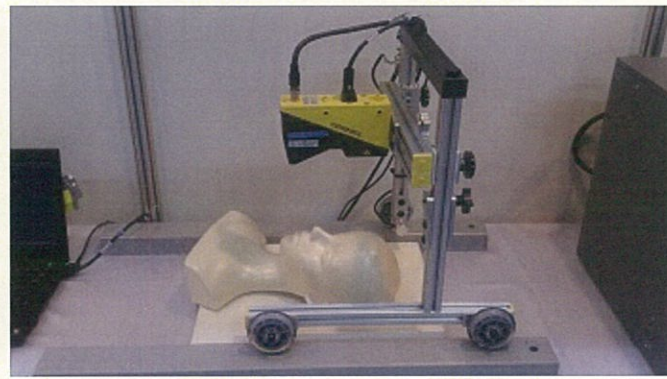
3Dセンサ DS1000 コグネックス(株)
